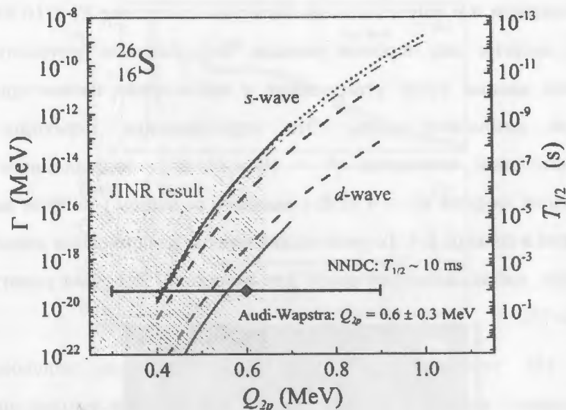
Рис.5. Расчёты границ ширины \Gamma и времени жизни T_{1/2} как функции энергии 2p -распада. Сплошные и пунктирные линии соответствуют расчётам по модели квазиклассической спонтанной эмиссии и трехчастичной модели " I^2 ", соответственно, детали описаны в работе [7]. Заштрихованная зона, как следствие анализа данных, исключает возможный диапазон значений Q_{2p} и T_{1/2} . Символом с ошибками обозначены ранее принятые значения Q_{2p} = 0.6 \pm 0.3 МэВ и T_{1/2} \sim 10 мс.
