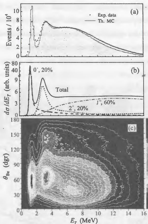
Рис.4. Спектр состояний {}^6\text{Be} : точки – эксперимент, гистограмма – результат симуляции методом Монте-Карло теоретической формы спектра с учётом эффективности установки (а). Результаты теоретических расчётов, которые послужили входными данными для МК-симуляций (б). Контурная диаграмма в координатах \theta_{\text{Be}}-E_T для данных, наблюдаемых в эксперименте (с).
