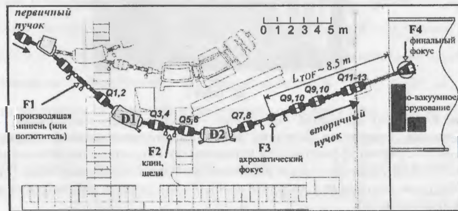
Рис.3. Верхняя панель: схема эксперимента по изучению {}^6\text{Be} в реакции {}^1\text{H}({}^6\text{Li}, {}^6\text{Be})n . Нижняя панель: установка АКУЛИНА, адаптированная для получения монохроматического первичного пучка {}^6\text{Li} нужной энергии. В плоскости F1 вместо производящей мишени устанавливался углеродный поглотитель энергии; в плоскости F2 зазор щелей составлял \pm 1.5 мм, клин не использовался.
