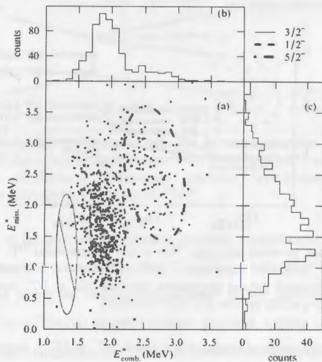
Рис. 8. Распределение событий тройных совпадений d-p-p в представлении E_{\text{emis}} - E_{\text{comb}} . События, локализованные в нижнем эллипсе с достоверностью 68%, взяты для определения верхнего предела соотношения \Gamma_{2p}/\Gamma_\gamma .
