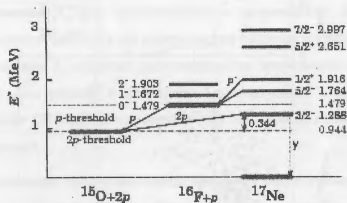
Рис.7. Схема уровней изотопа ^{17}\text{Ne} и его подсистемы ^{16}\text{F} . Стрелками показаны способы распада возбуждённых состояний ^{17}\text{Ne} : последовательный распад протонами уровней 5/2^+ и 1/2^+ , испускание \gamma -квантов и 2p -распад уровня 3/2^- ( E = 1288 кэВ).
